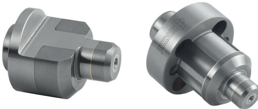
Flanschaufnahme mit vollen und abgeflachten Hartmetall-Ringen
